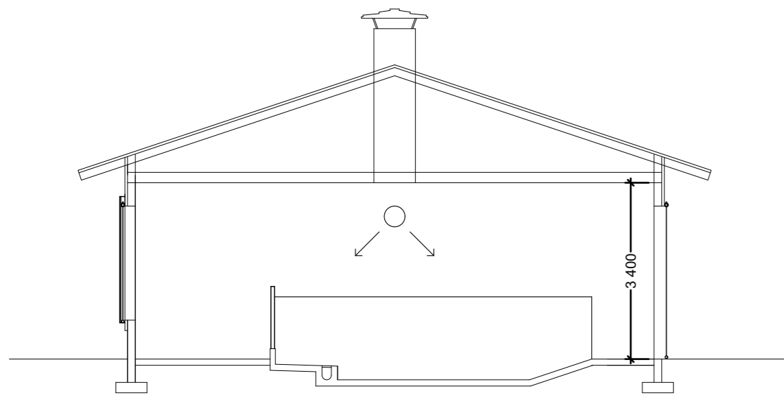
LEIKKAUS A-A
