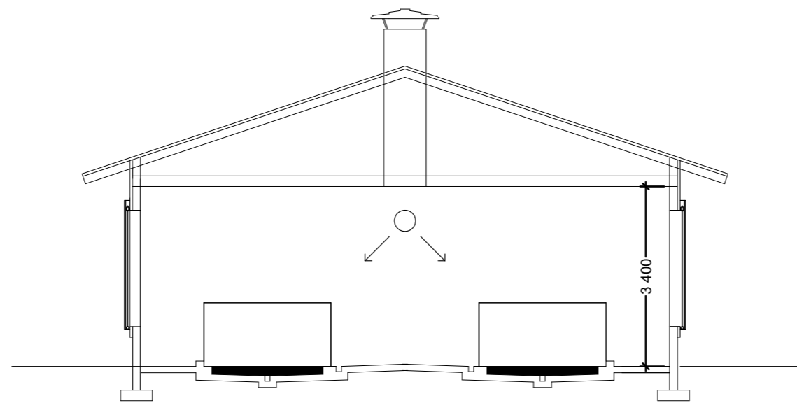
LEIKKAUS B-B
