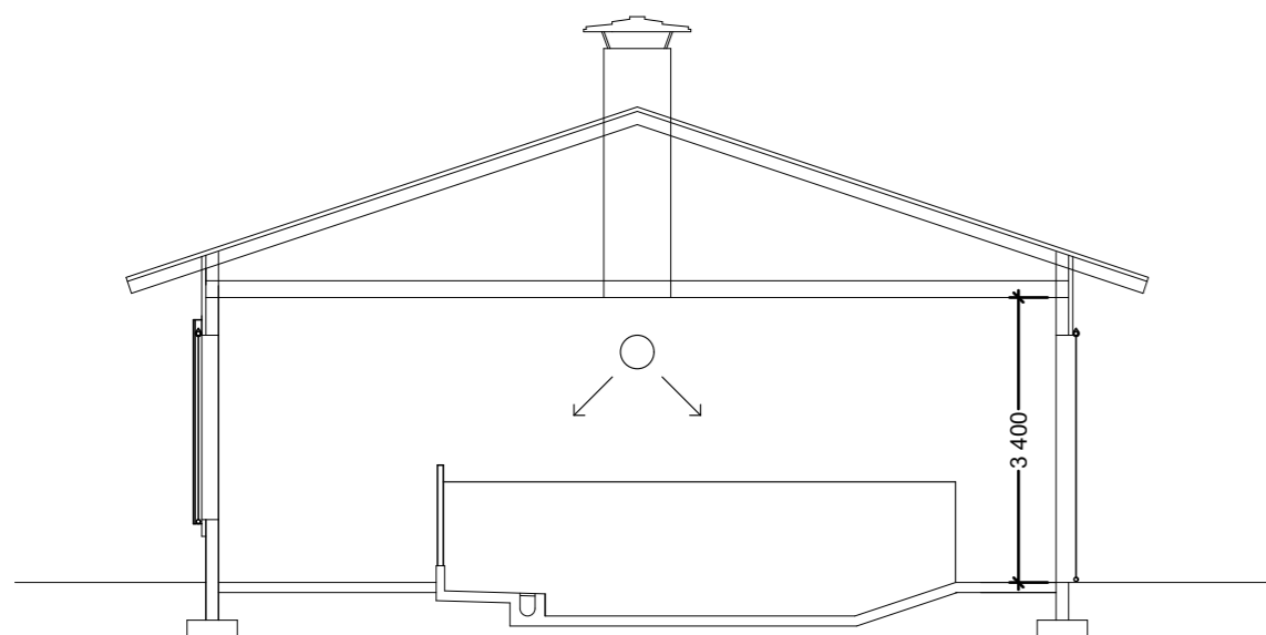
LEIKKAUS A-A
