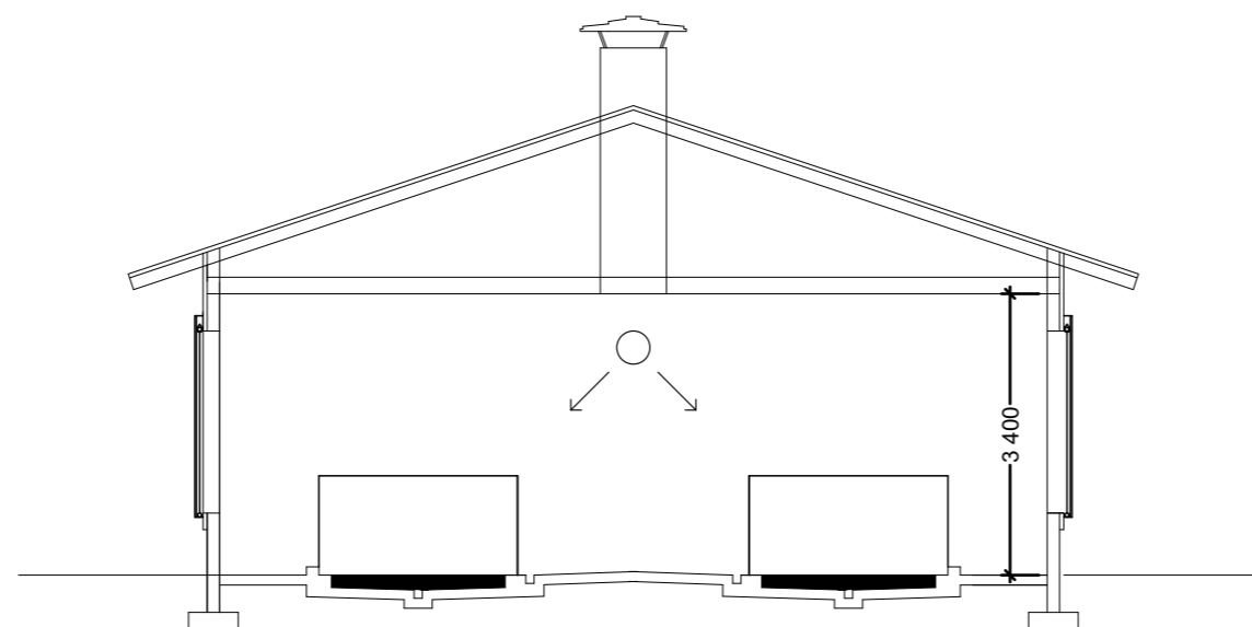
LEIKKAUS B-B
