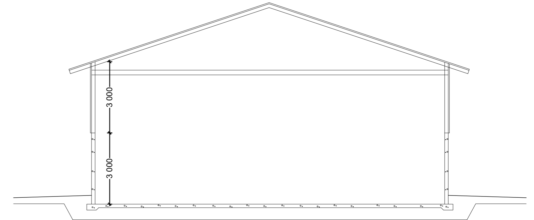
LEIKKAUS LANTALASTA
