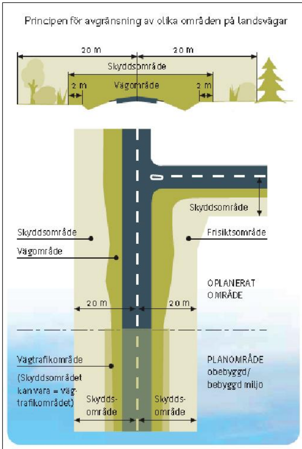
Bild 1. Principen för avgränsning av olika områden på landsvägar ( https://www.elv-keskus.fi/sv/web/elv/suoja-ja-nakemaalueelle-rakentaminen?p_p_id=122_INSTANCE_aluevalinta&p_p_lifecycle=0&p_p_state=normal&p_p_mode=view&p_r_p_564233524_resetCursor=true&p_r_p_564233524_categoryId=14405#.WIYVofll-Uk )
